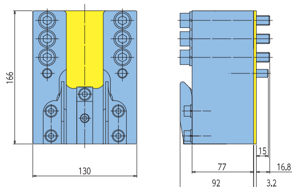
CBCBK-150-640-P-A2(ストッパプレート付)
