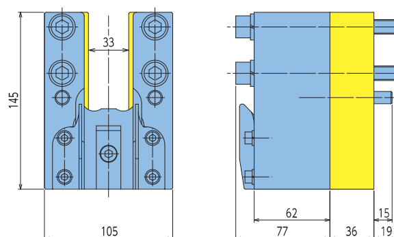
CBCBK-100-550-W-A2 (配管スペース付)
