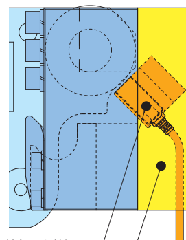
バー検知用近接SW 近接SW取付ブロック
