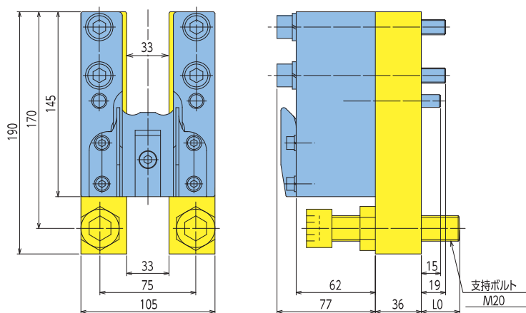
CBCBK-100-550-LO-A2(支持ボルト付)
