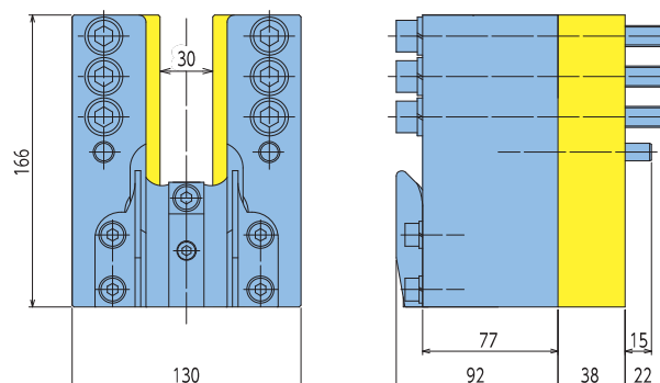
CBCBK-150-640-W-A2 (配管スぺーサ付)
