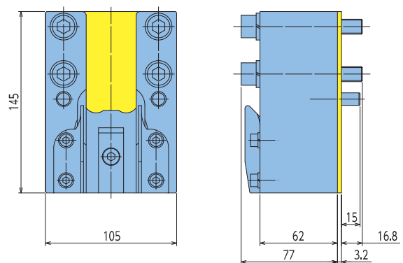
CBCBK-100-550-P-A2(ストッパプレート付)
