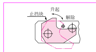
止挡块动作原理图
