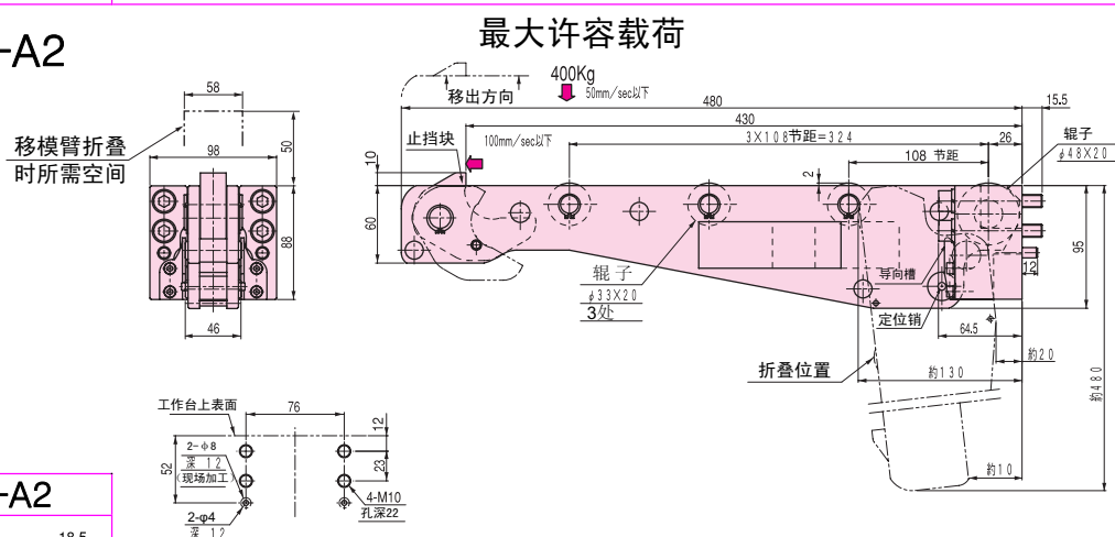
安装尺寸 辊子高出工作台面2mm
