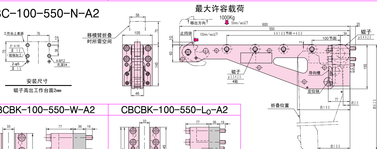
安装尺寸 辊子高出工作台面2mm
